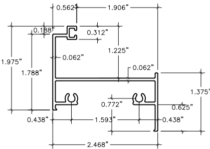
2 FRAME JAMB
